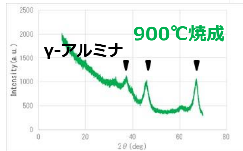
図.X線回折
