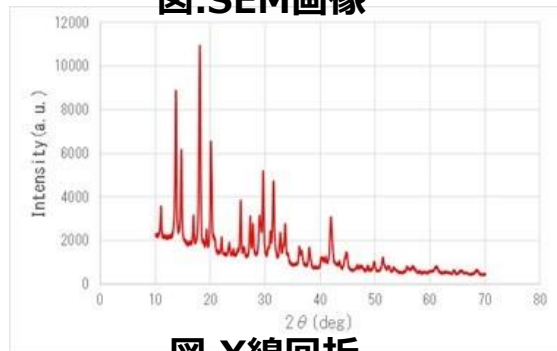
図.X線回折
