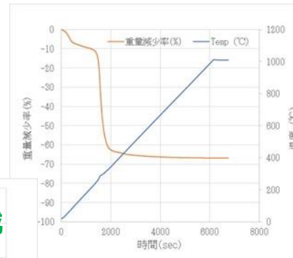
図.TG-DTA
